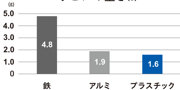
ボビンの重さ(g)
