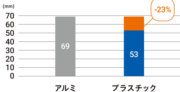
糸切り後のボビンケース内部のたわみ糸量
