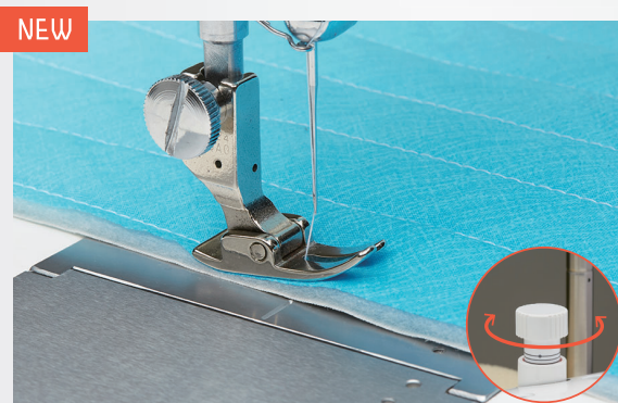
NEW フロート機能（微量押え上げ）
