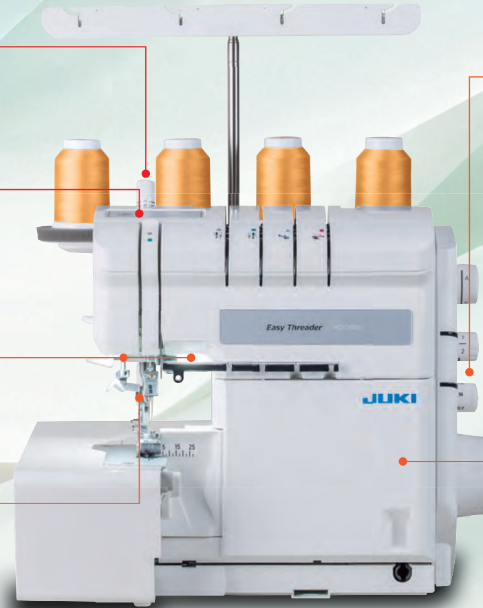
上: 縫い目長さ調節つまみ 下: 差動調節つまみ
