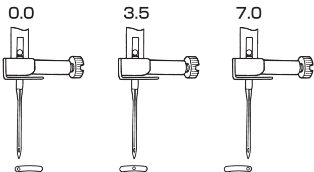
調節ダイヤル（左）
