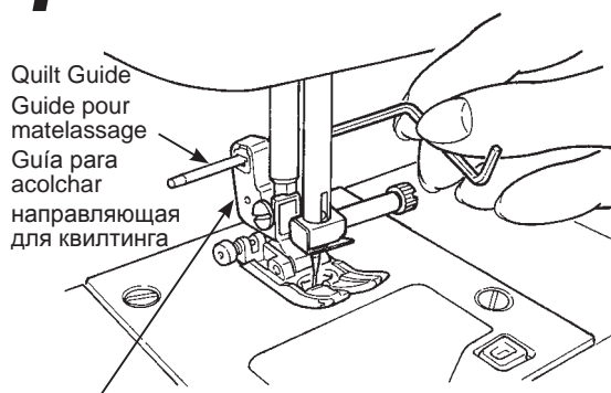
Presser foot holder Support pied presseur Soporte del prensatelas держатель прижимной лапки
